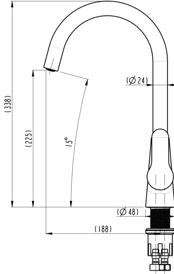
BE11042106 Bien Capri Konik Eviye Bataryası ( U borulu )
