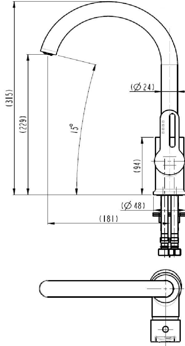
BE11050105 Bien Jenny Round Eviye Bataryası (U Borulu)
