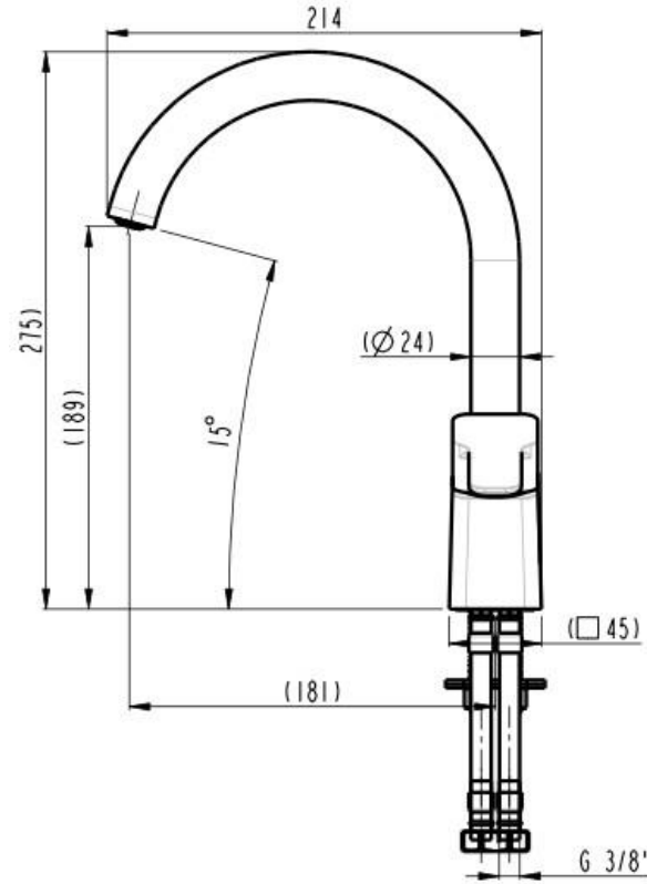
BE11062103 Bien Goya Eviye Bataryası (U borulu)
