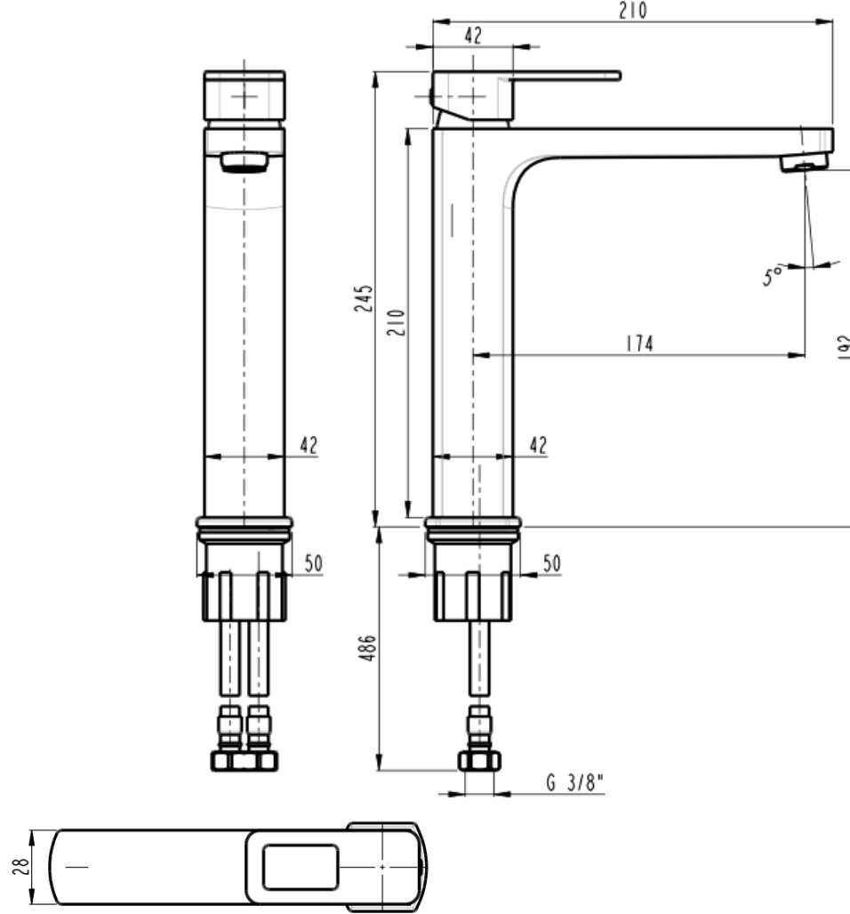
BL21065415 Bien Salvo Plus Colours Orta Boy Yüksek Tip Lavabo Bataryası - Beyaz -Rose Gold
