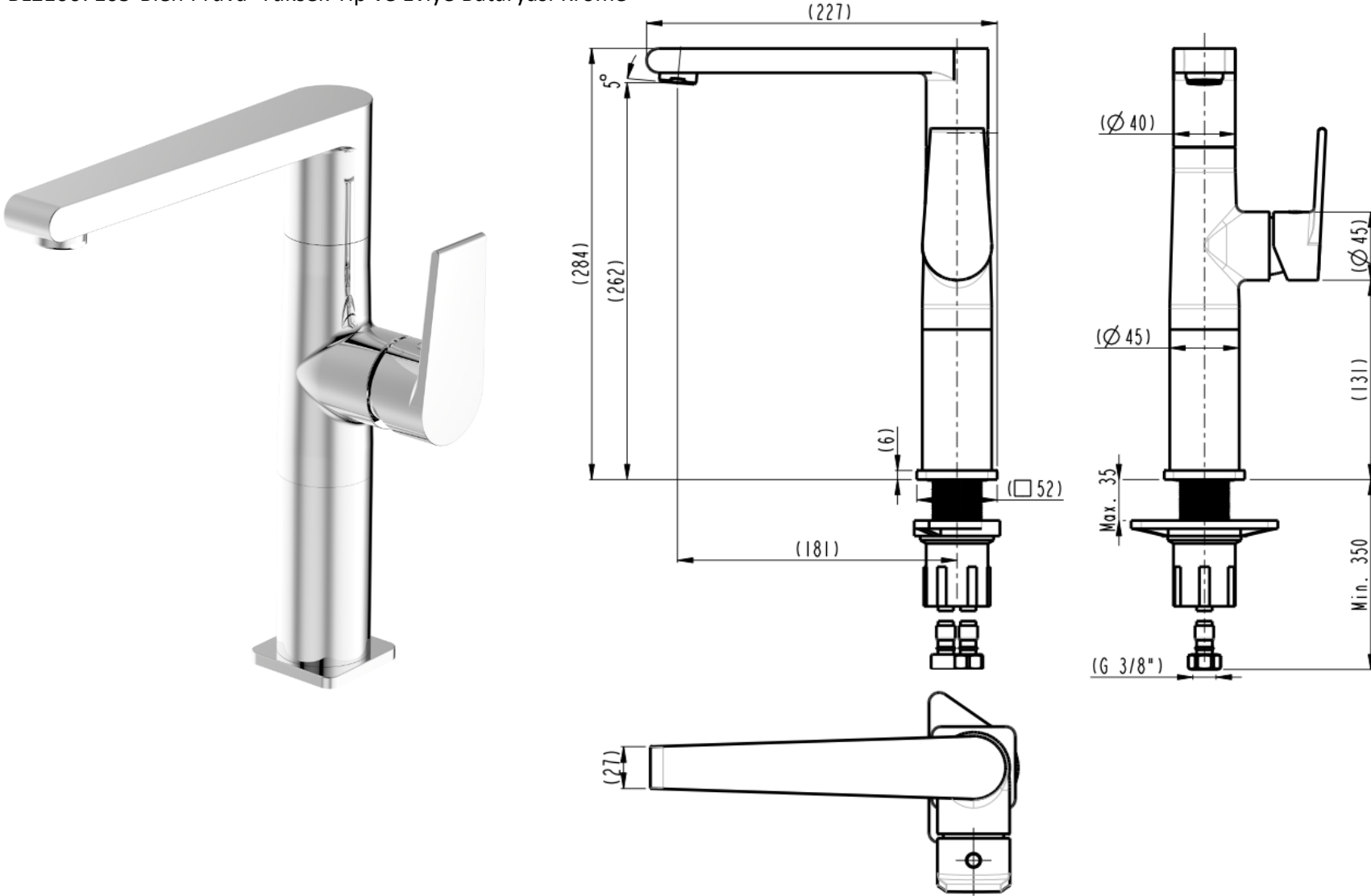
BL21067105 Bien Pruva Yüksek Tip ve Eviye Bataryası Krome
