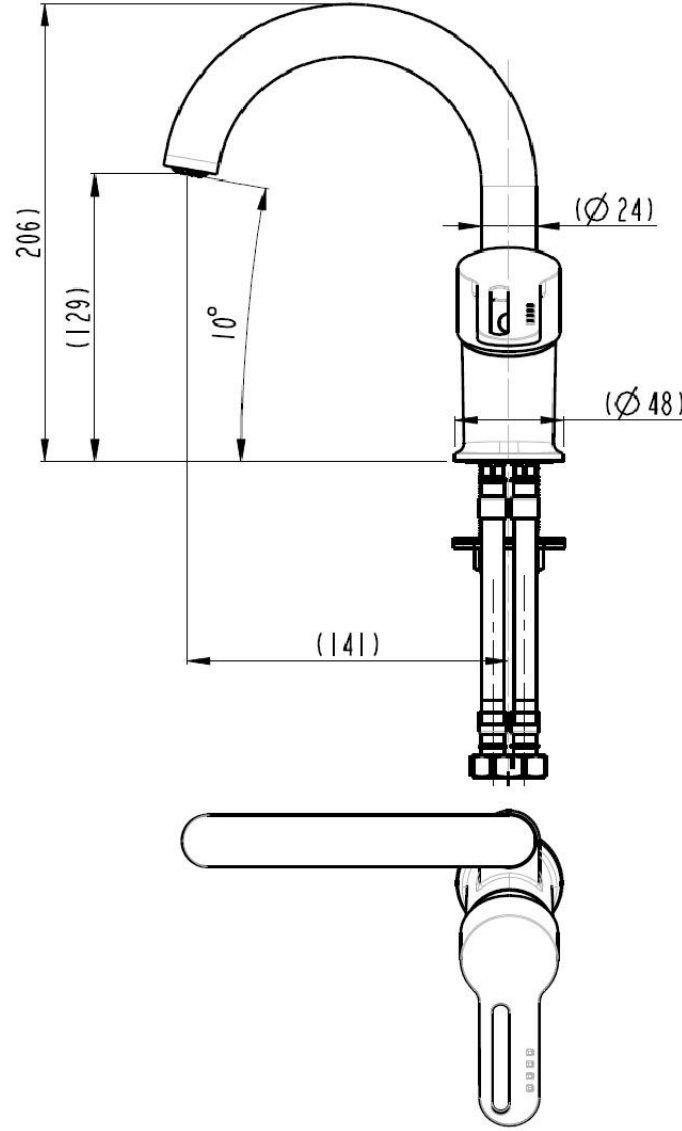
BL31050104 Bien Jenny Lavabo Bataryası (U Borulu)
